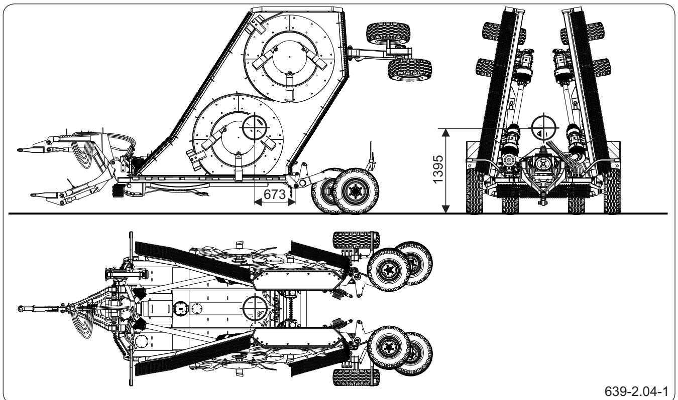
Rysunek 2.5 Położenie środka ciężkości maszyny
