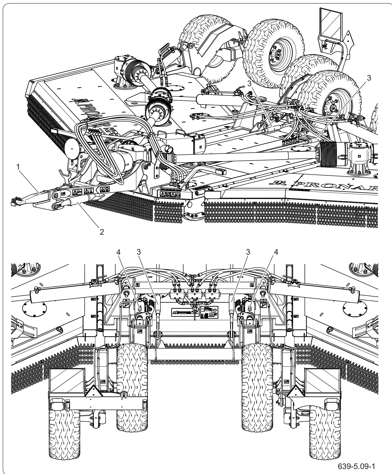
Rysunek 5.5 Regulacja położenia maszyny
