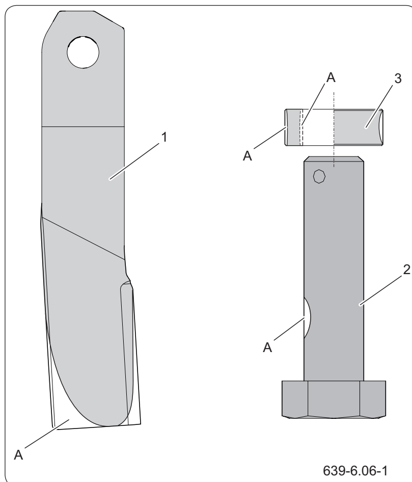
Rysunek 6.12 Potencjalne miejsca zużycia elementów głowicy
