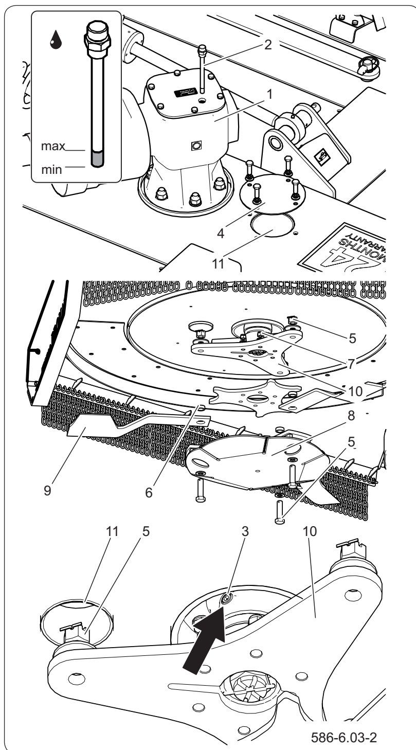
Rysunek 6.10 Kontrola i wymiana oleju w przekładniach kątowych
