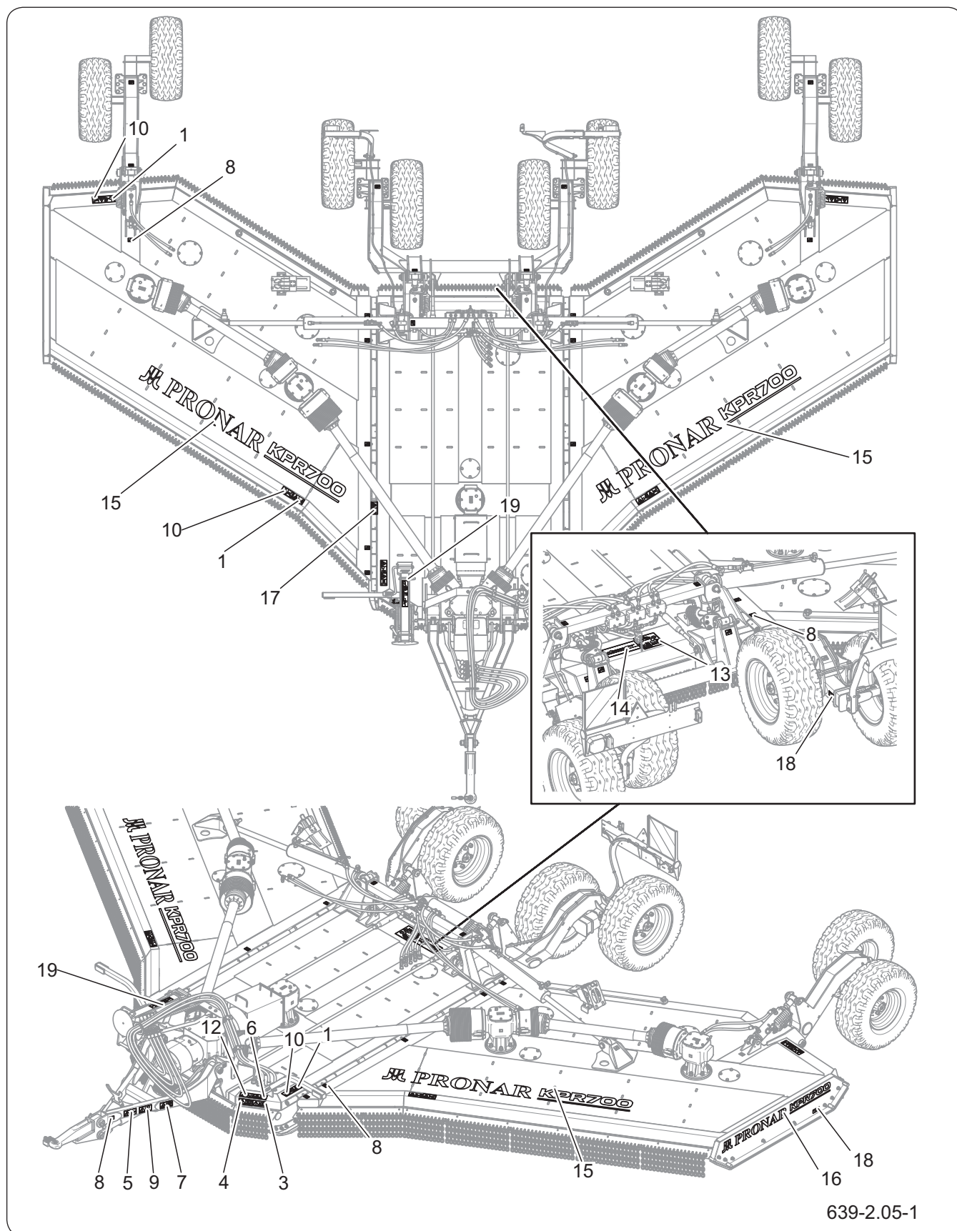
Rysunek 3.1 Rozmieszczenie nalepek informacyjnych i ostrzegawczych
