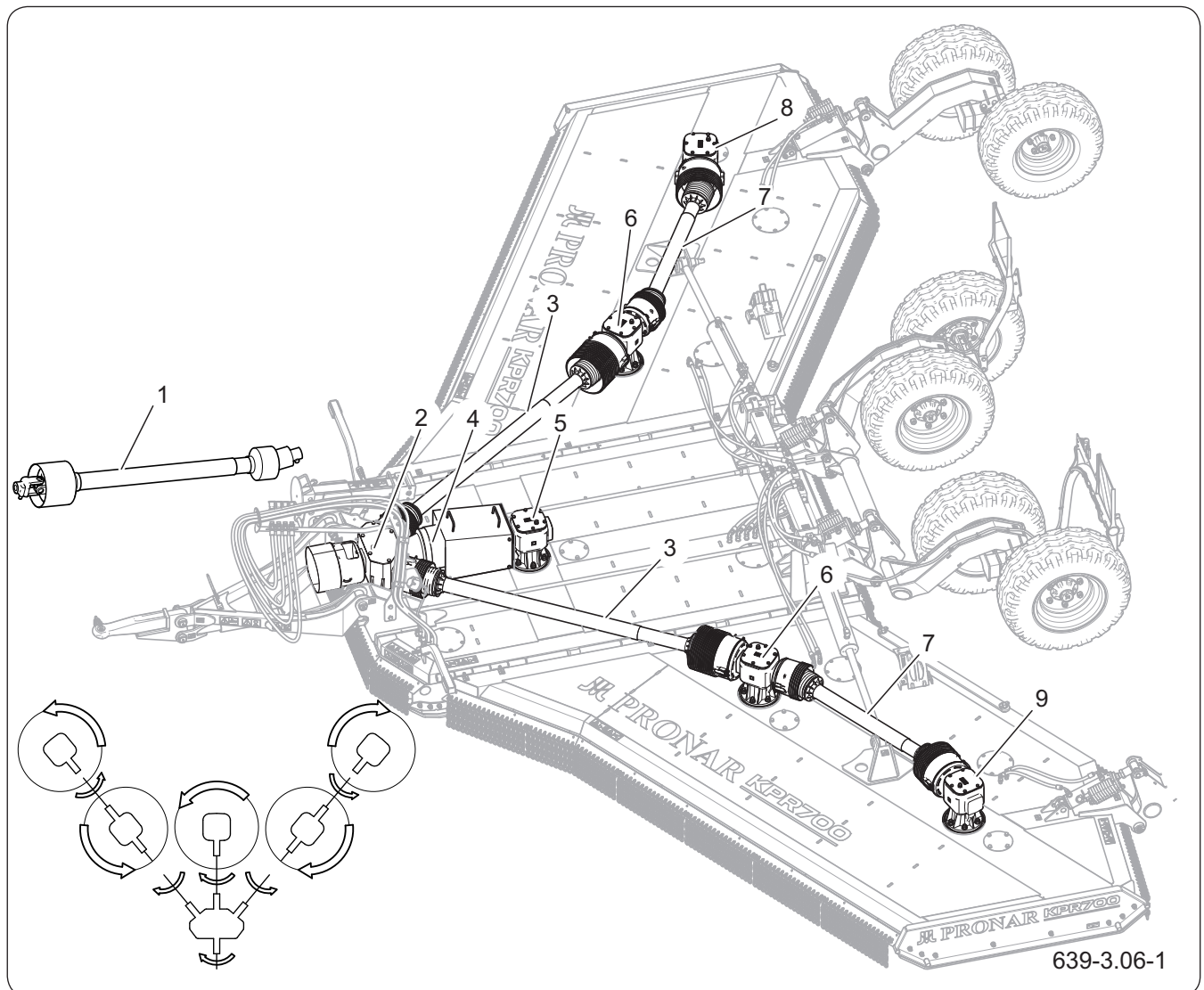
Rysunek 4.5 Budowa układu napędowego kosiarki KPR700
