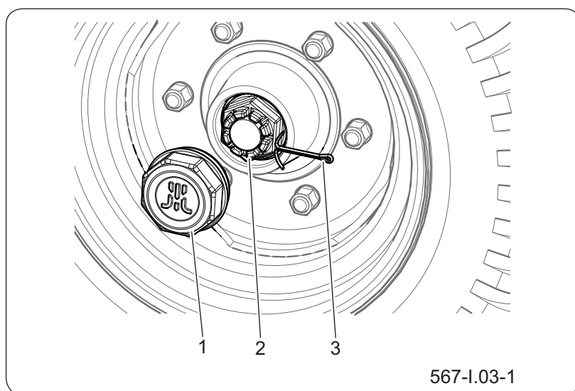
Rysunek 6.7 Regulacja luzu łożysk osi jezdnej
