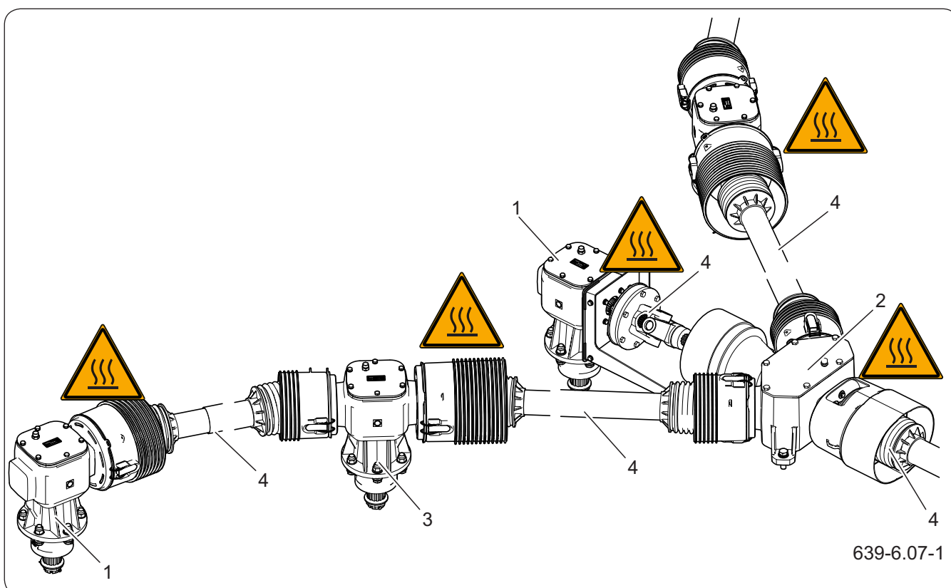
Rysunek 6.8 Kontrola i wymiana oleju w przekładni
