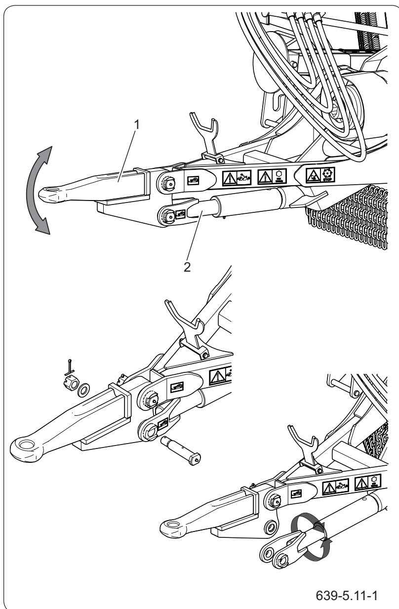
Rysunek 5.6 Ustawienie pochylenia dyszla
