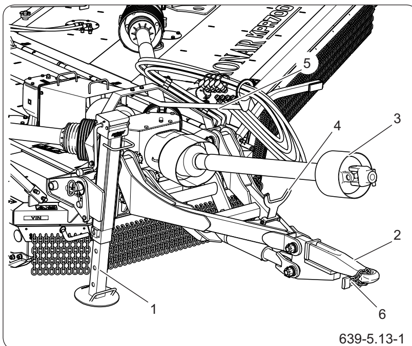
Rysunek 5.8 Łączenie kosiarki z nośnikiem
