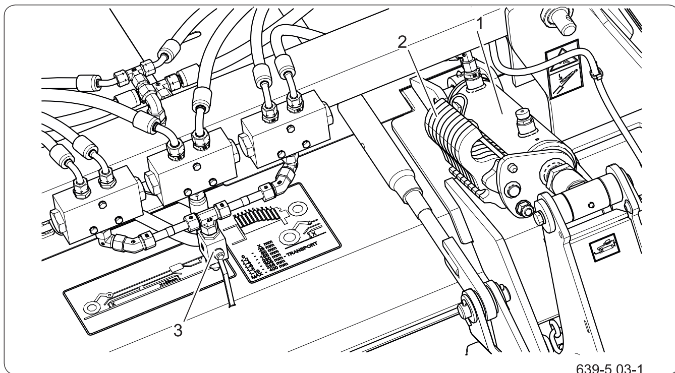
Rysunek 5.10 Blokady transportowe II
