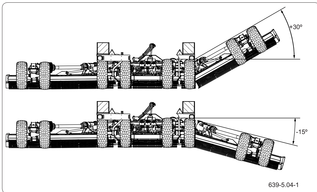
Rysunek 5.11 Praca kosiarką na pochyłości - kopiowanie terenu
