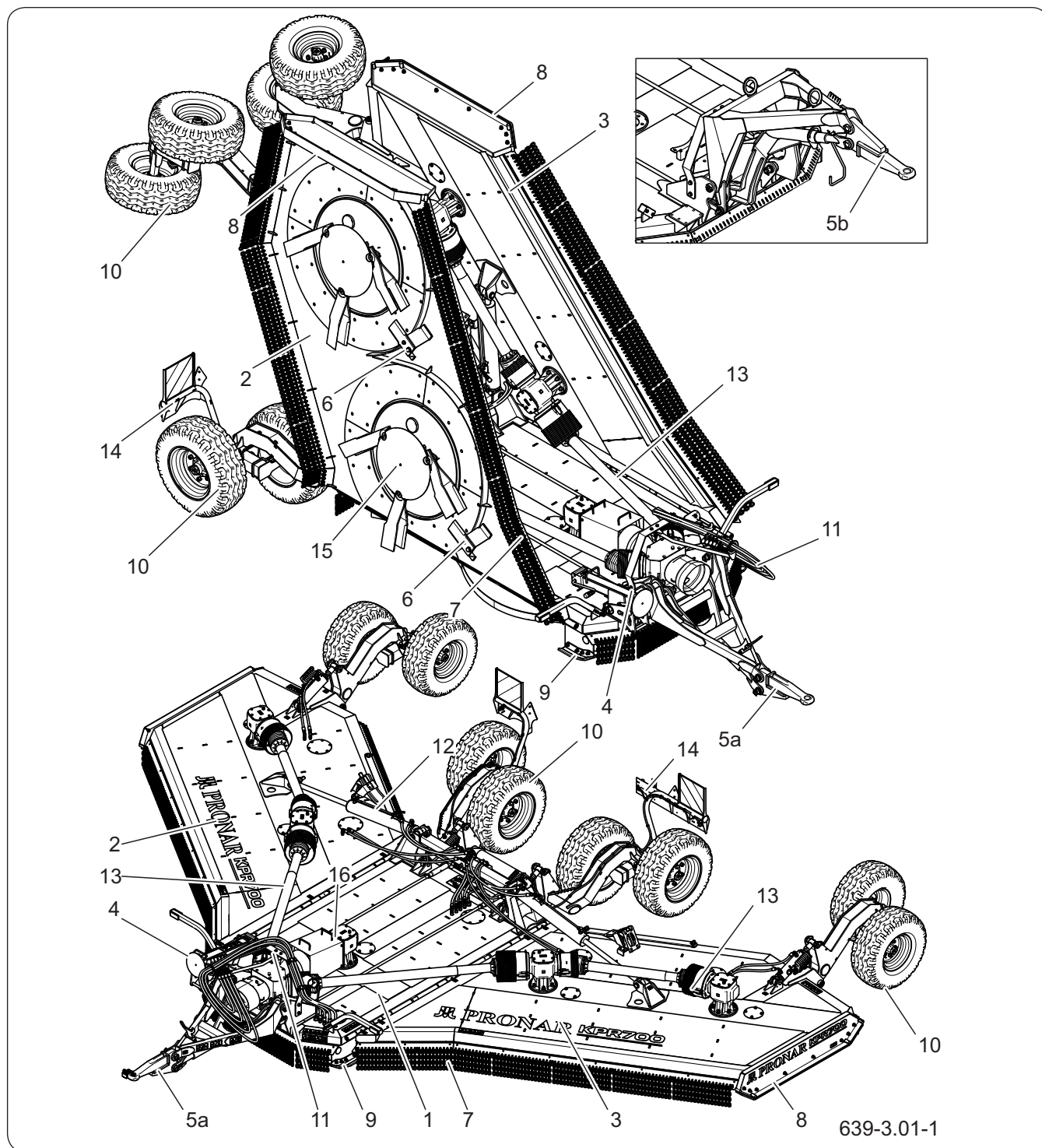
Rysunek 4.1 Budowa maszyny
