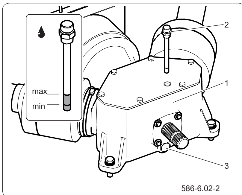
Rysunek 6.9 Kontrola i wymiana oleju w przekładni rozdzielającej
