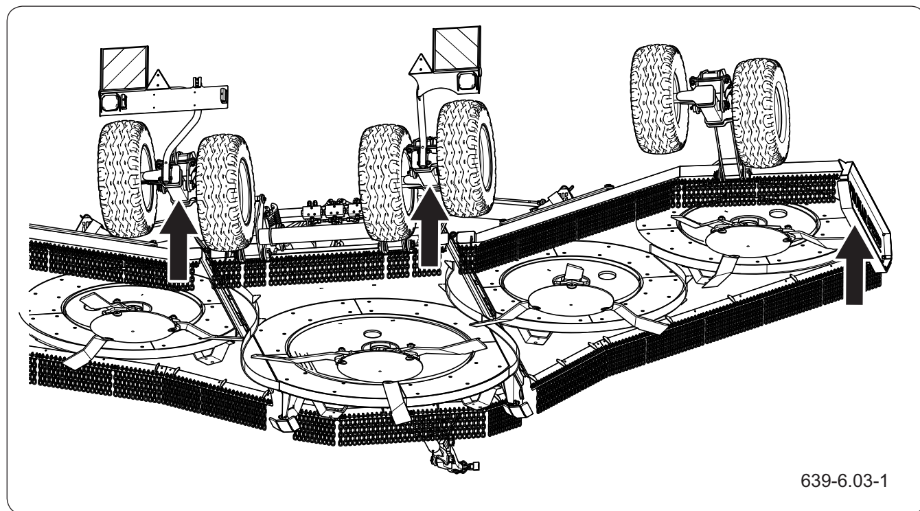
Rysunek 6.5 Punkty podparcia podnośnika
